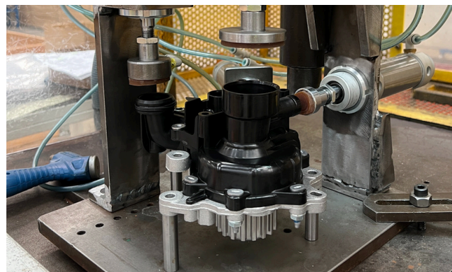
N210CT TEST DE FUGA DE LA BOMBA INSTALACIONES DOLZ (ESPAÑA)
