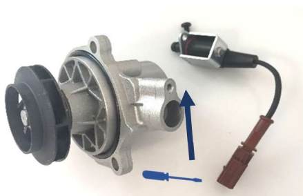
Waterpump A255 (mechanical versión)
